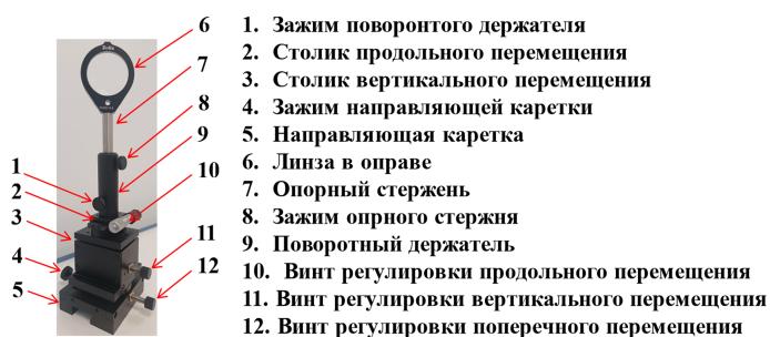
Рис. IV. Рейтер трёхкоординатный
